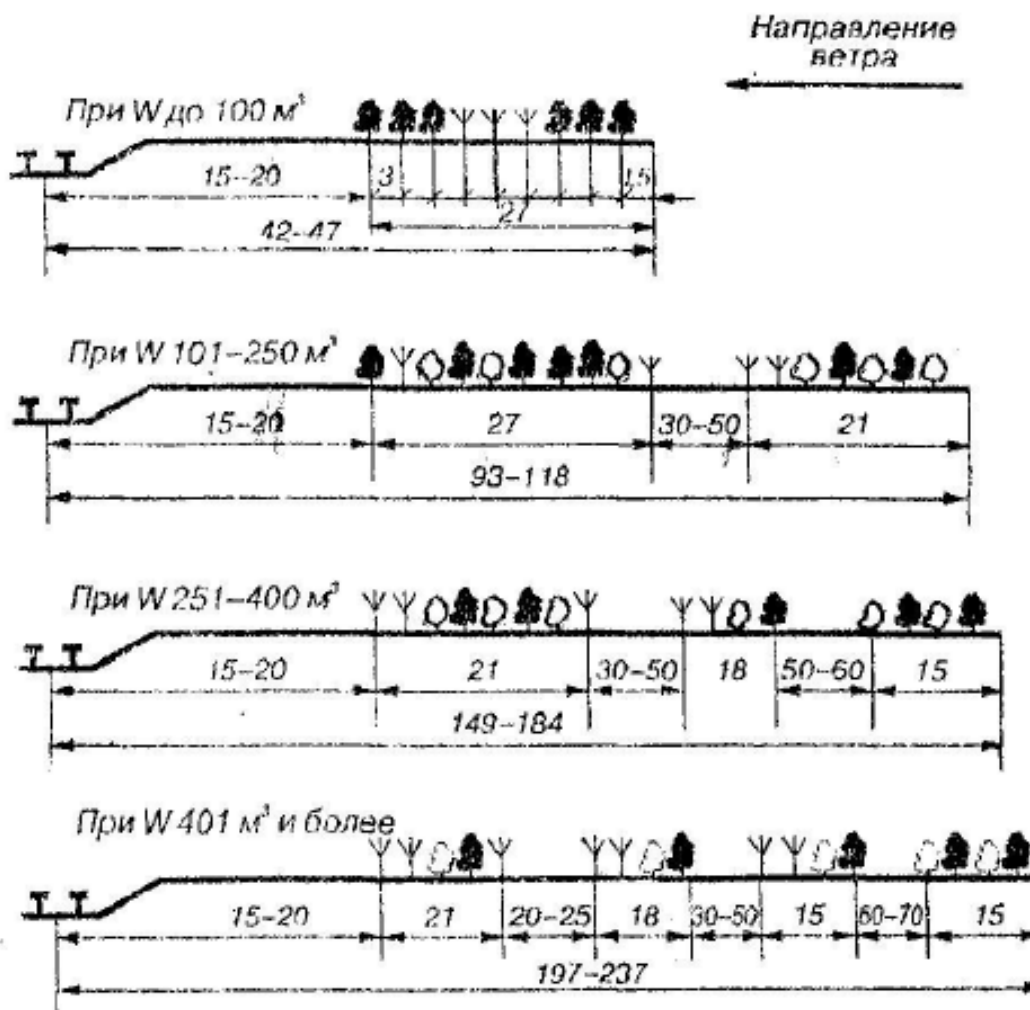
Рисунок 1 - Схемы снегозадерживающих лесных полос вдоль железных дорог Размещение снегозадерживающих лесных полос вдоль полотна железной дороги, асор-
